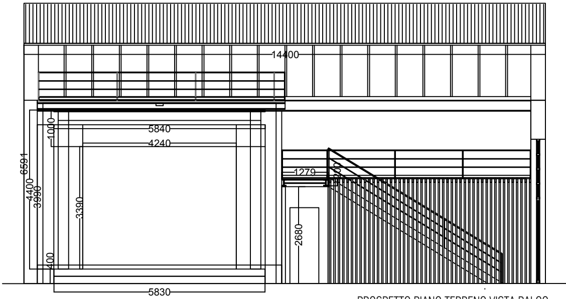
PROSPETTO PIANO TERRENO VISTA PALCO
